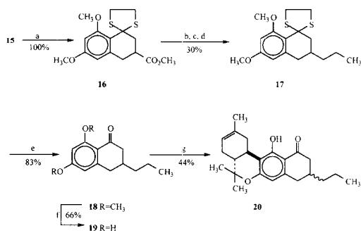
Scheme 2. (a) HSCH 2 CH 2 SH/BF 3 ·Et 2 O/CH 2 Cl 2 /25 °C; (b) LiAlH 4 /THF/25 °C; (c) TsCl/C 6 H 5 N/CHCl 3 /0 °C; (d) EtMgBr/Li 2 CuCl 4 /THF/25 °C; (e) CH 3 I/CH 3 OH/H 2 O/reflux; (f) BBr 3 /CH 2 Cl 2 /25 °C; (g) trans - p -menthadienol/HOTs/C 6 H 5 F/reflux.
