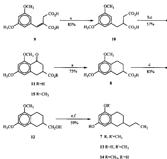
Scheme 1. (a) H 2 (g)/10% Pd(C)/EtOH/48 psi; (b) Ac 2 O/reflux; (c) PPA/100 °C; (d) LiAlH 4 /THF/25 °C; (e) TsCl/C 5 H 5 N/CHCl 3 /0 °C; (f) EtMgBr/Li 2 CuCl 4 /THF/25 °C.
